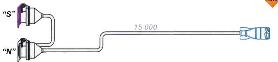
FA102706-DL Cableado delantero
