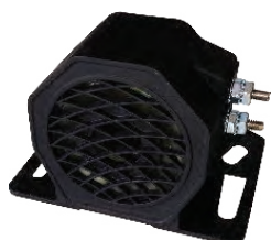
VG630120 12/24 V 87 dB
