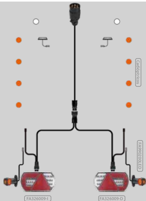
FA328008 KIT REMOLQUE CON PILOTOS CON TRIÁNGULO Y POSICIÓN DE ANCHURA Pag. 319
